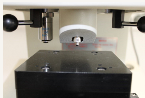
Detalle de punta de microindentador
