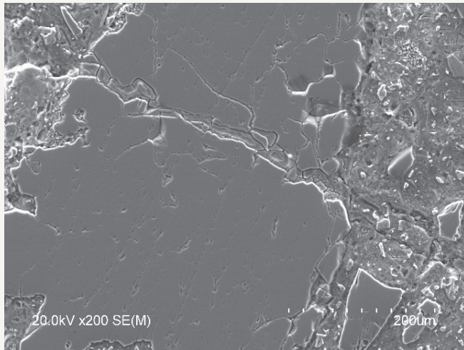
Hormigón con árido silíceo y productos de reacción RAS fisurando el árido con geles
