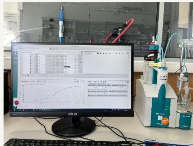
Equipo de valoración potenciométrica con resultados en la pantalla del controlador
