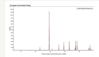
Espectro de difracción de rayos X del \text{CaCO}_3
