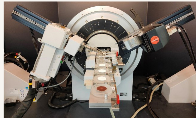
Detalle del goniómetro del carrusel de muestras
