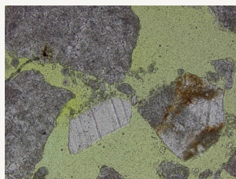
(4x [X]). Fragmentos de dolomías
