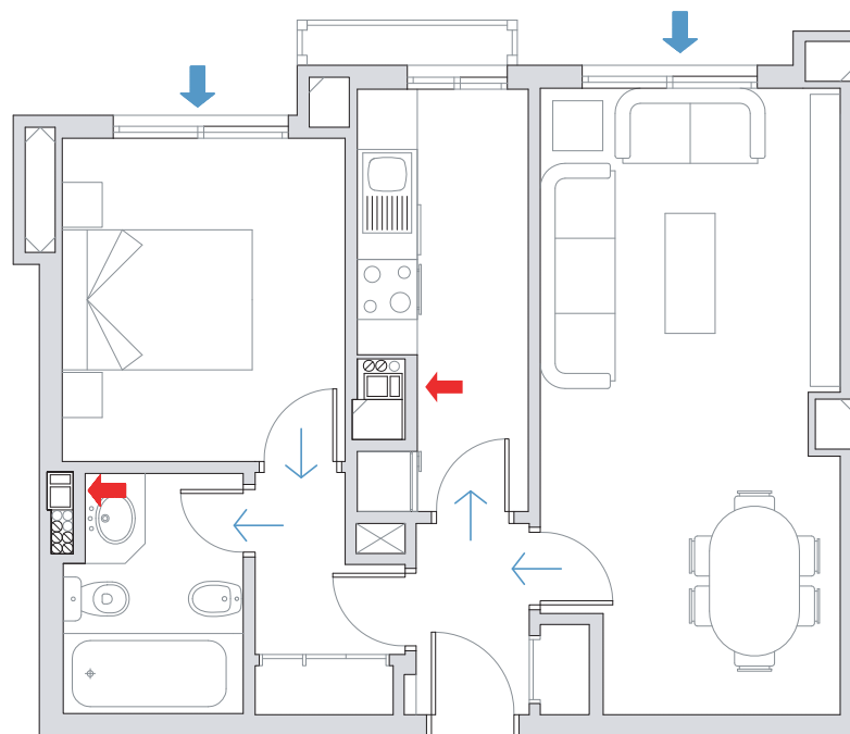
Figura 3.10.1 Planta de una de las viviendas
