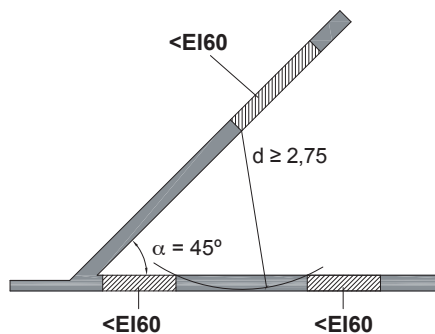
DB SI 2 Figura 1.2 Fachadas a 45°
