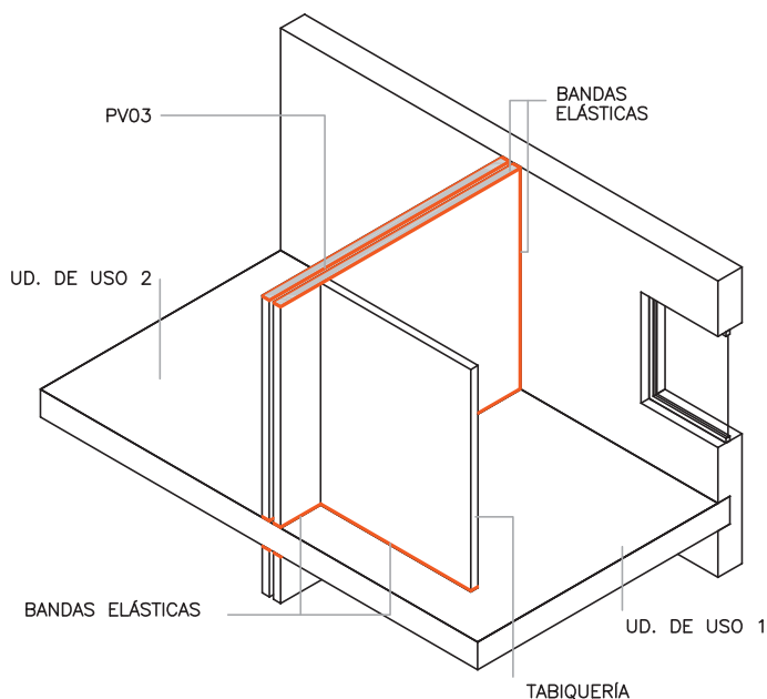
Figura 4.3. Encuentros de particiones de tipo PV03
