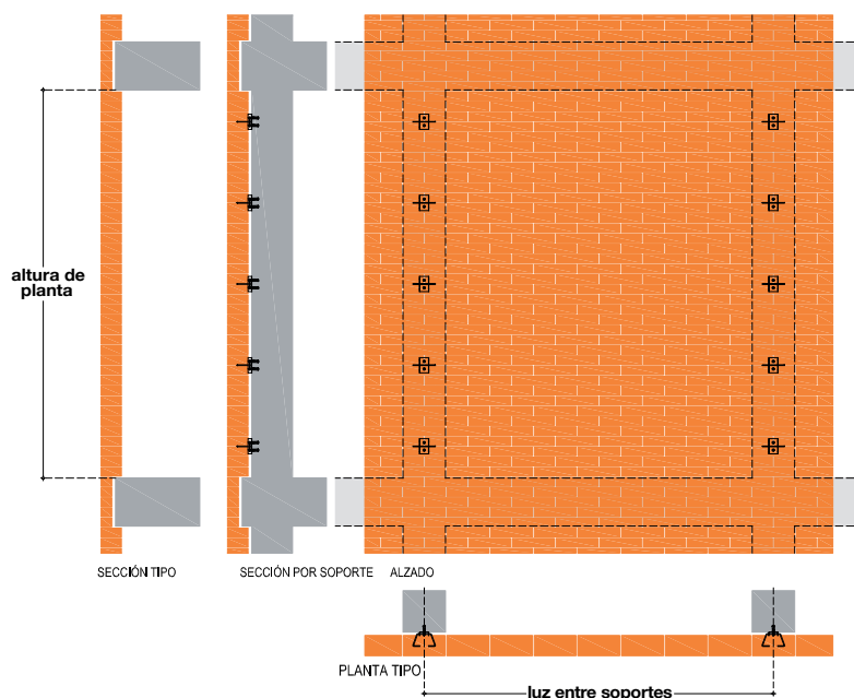
Figura A.1. Esquema de cerramiento sustentado en forjados y soportes
