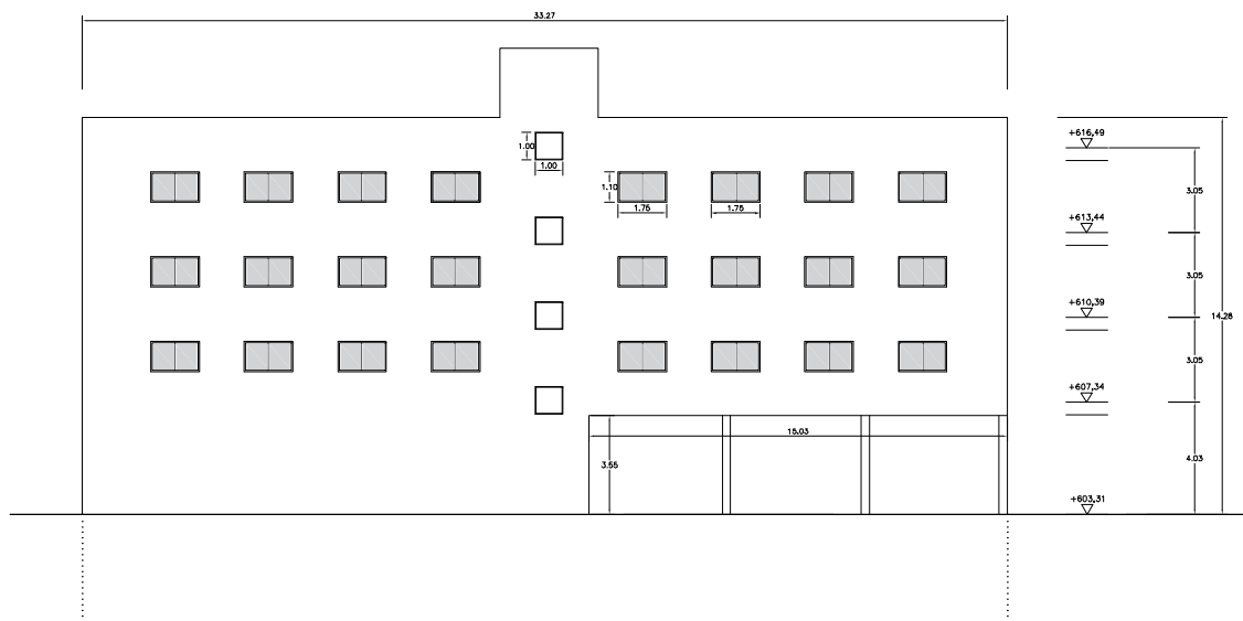
Figura 5.7 Alzado norte
