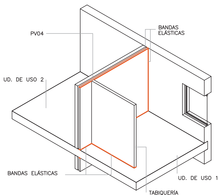
Figura 4.4. Encuentros de particiones de tipo PV04
