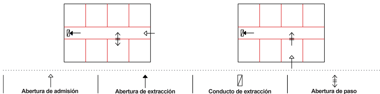
DB HS 3 Figura 3.2 Ejemplos de tipos de ventilación en trasteros
