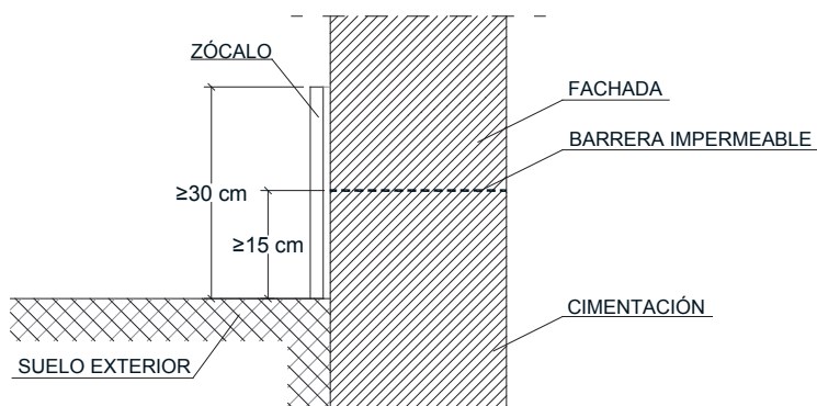
DB HS 1 Figura 2.7 Ejemplo de arranque de la fachada desde la cimentación
