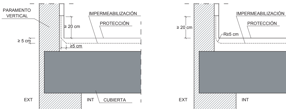
DB HS 1 Figura 2.13 Encuentro de la cubierta con un paramento vertical
