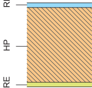
FC07: Una hoja, hoja principal de 1 pie, revestimiento continuo
