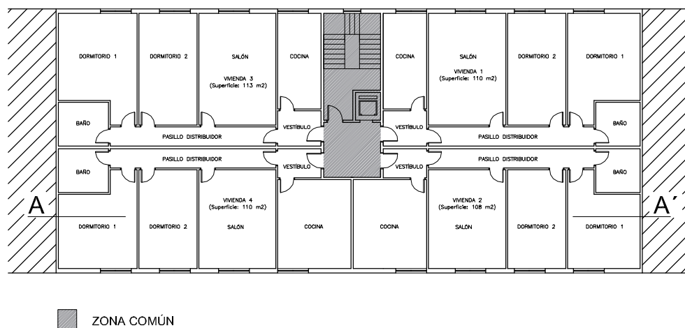
Figura 5.3 Planta tipo
