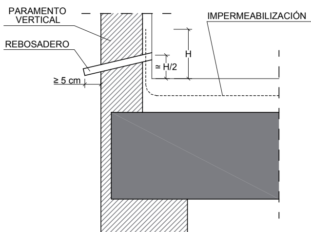
DB HS 1 Figura 2.15 Rebosadero
