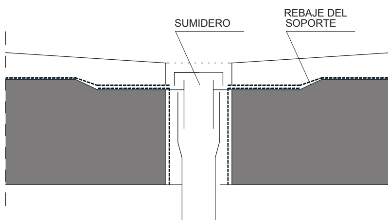
DB HS 1 Figura 2.14 Rebaje del soporte alrededor de los sumideros
