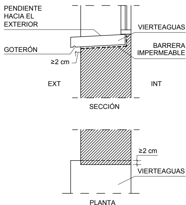
DB HS 1 Figura 2.12 Ejemplo de vierteaguas
