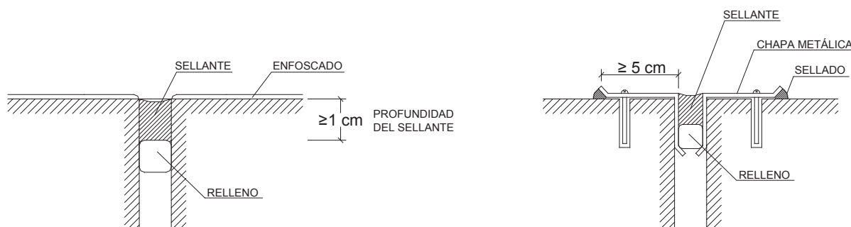
DB HS 1 Figura 2.6 Ejemplos de juntas de dilatación
