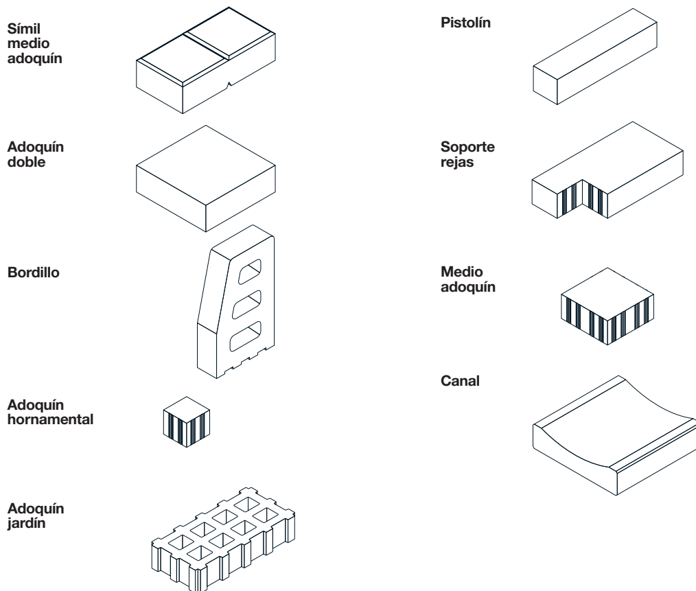
Figura 2.20 Piezas especiales adoquín cerámico
