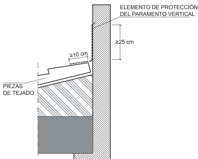
DB HS 1 Figura 2.16 Encuentro en la parte superior del faldón
