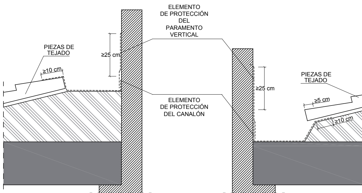
DB HS 1 Figura 2.17 Canalones
