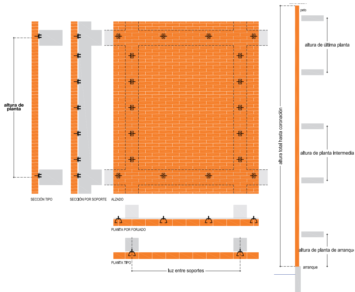
Figura A.2. Esquema de cerramiento autoportante
