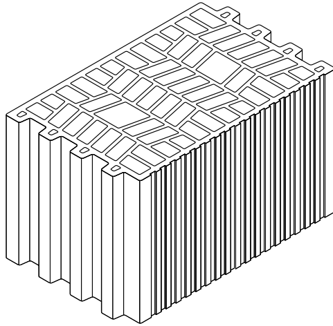
Figura 2.7 Bloques cerámico aligerado machihembrado
