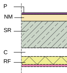
Figura 3.4.1 Falso techo
