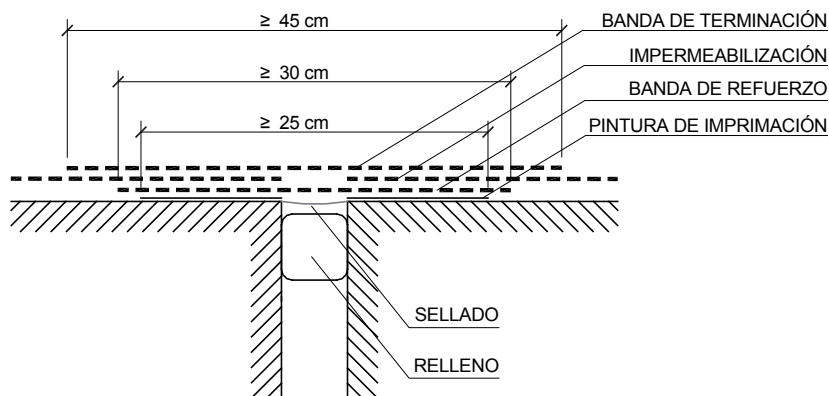
DB HS 1 Figura 2.2 Ejemplo de junta estructural
