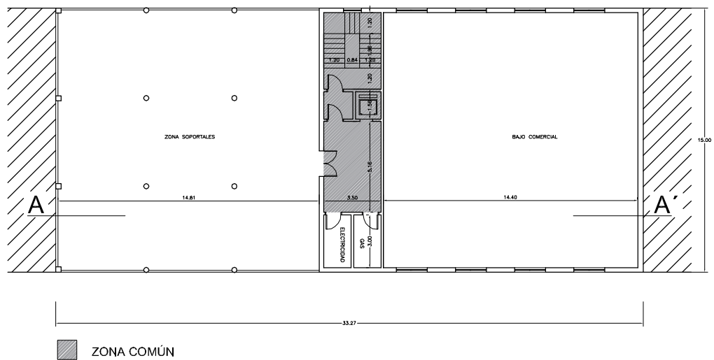
Figura 5.3 Planta tipo
