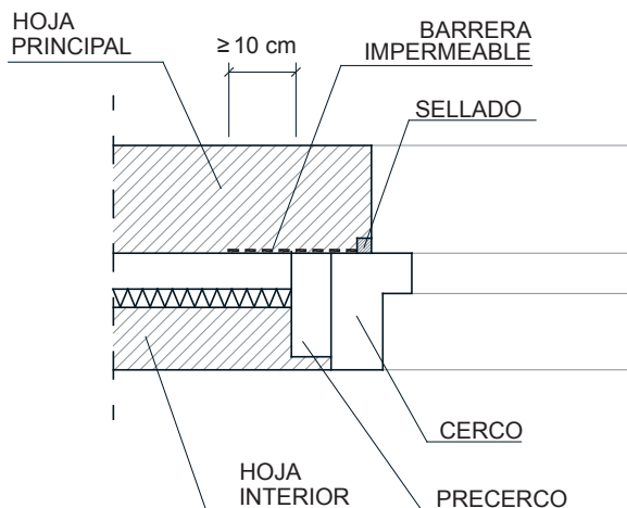
DB HS 1 Figura 2.11 Ejemplo de encuentro de la fachada con la carpintería
