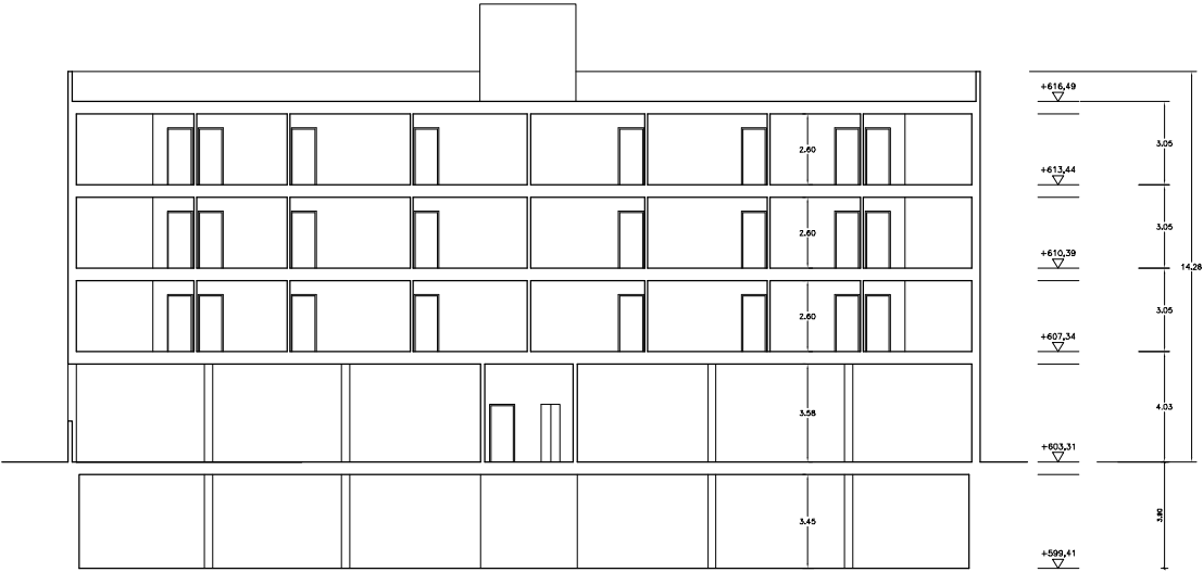
Figura 5.4 Sección A-A'
