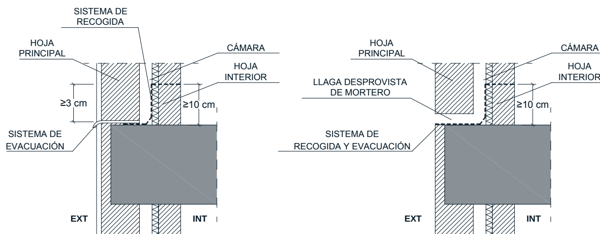
DB HS 1 Figura 2.10 Ejemplo de encuentro de la cámara con los forjados
