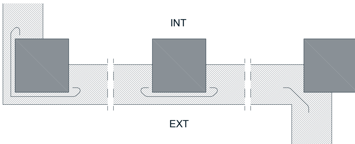
DB HS 1 Figura 2.9 Ejemplo de encuentro de la fachada con los pilares
