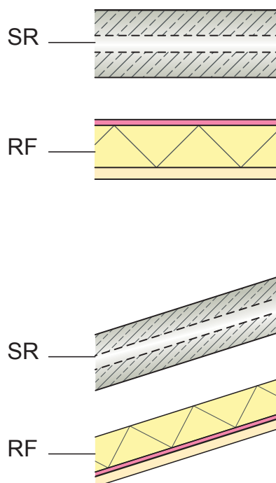
Figura 3.5.1 Falsos techos
