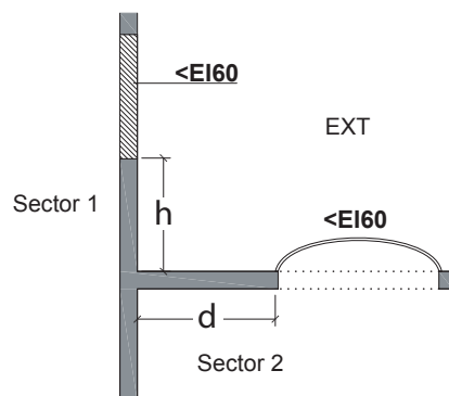
DB SI 2 Figura 2.1 Encuentro cubierta-fachada
