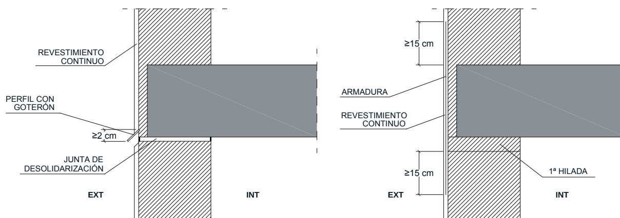
DB HS 1 Figura 2.8 Ejemplos de encuentros de la fachada con los forjados
