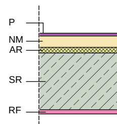
Figura 3.4.2 Aislante a ruido de impacto
