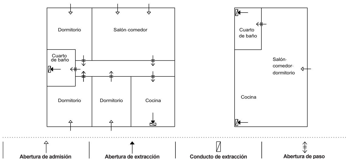
DB HS 3 Figura 3.1 Ejemplos de ventilación en el interior de las viviendas
