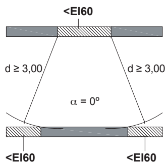
DB SI 2 Figura 1.1 Fachadas enfrentadas
