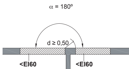
DB SI 2 Figura 1.6 Fachadas a 180°
