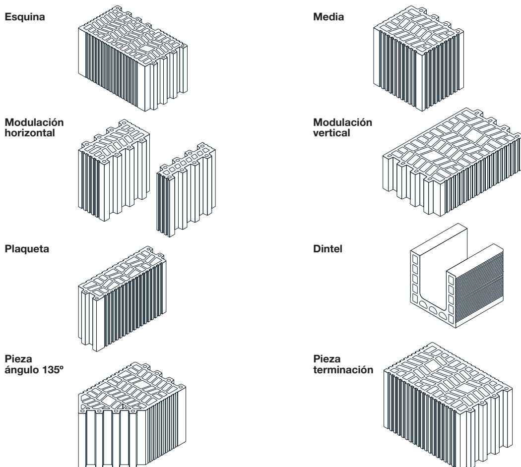
Figura 2.11 Piezas especiales bloque cerámico machihembrado
