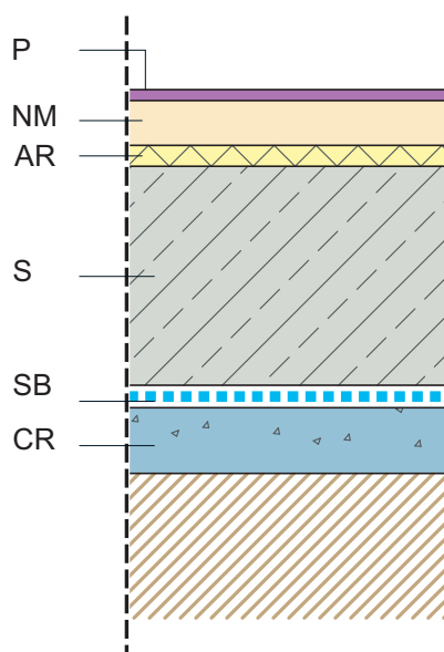
Figura 3.7.1 Aislante a ruido de impacto
