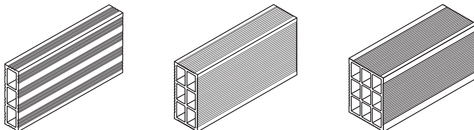
Figura 2.4 Ladrillos huecos para revestir (sencillo, doble y triple)
