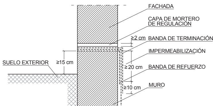
DB HS 1 Figura 2.1 Ejemplo de encuentro de un muro impermeabilizado por el interior con lámina con una fachada
