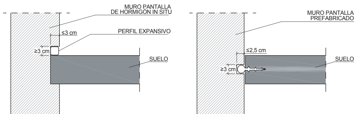
DB HS 1 Figura 2.3 Ejemplos de encuentro del suelo con un muro
