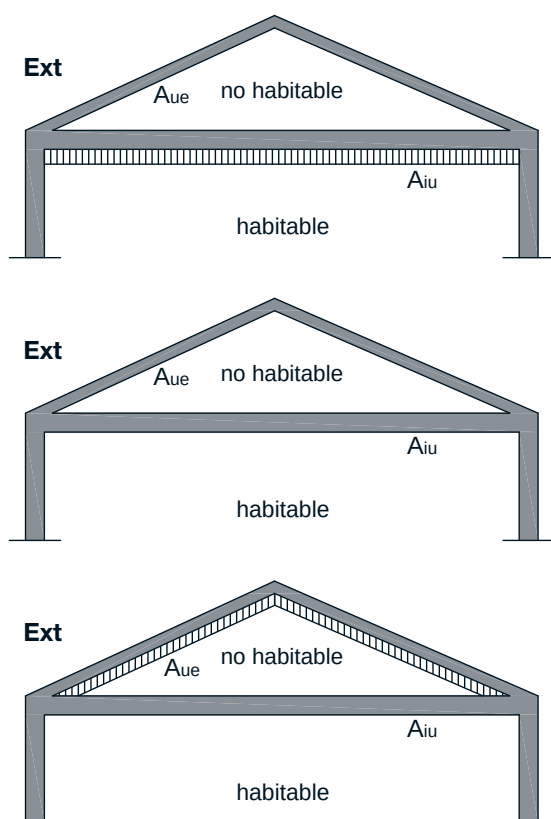
DB HE 1 Figura E.6 Espacios habitables en contacto con espacios no habitables
