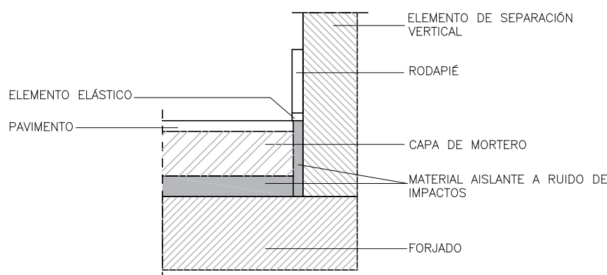
Figura 4.8. Vista en sección de un encuentro suelo flotante con una partición vertical
