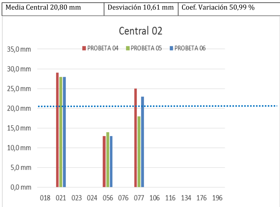
Gráfica 6.2. Laboratorios participantes, por Central con datos de Profundidad Máxima
