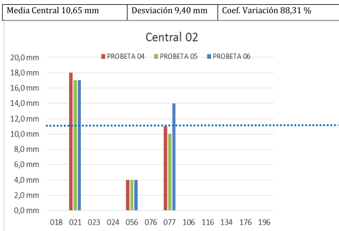
Gráfica 6.1. Laboratorios participantes, por Central con datos de Profundidad Media
