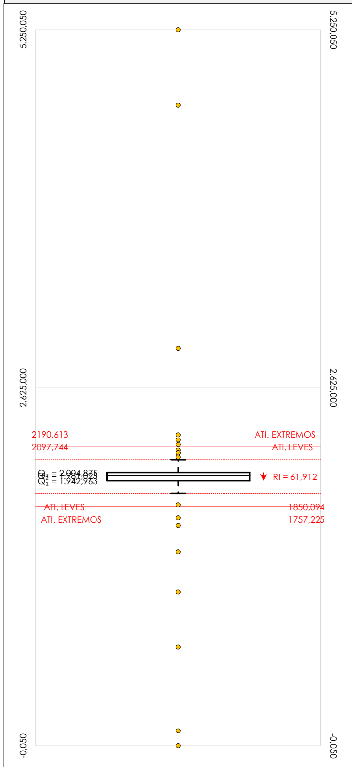
Diagrama Box-Plot pre-estadístico. Eje Y: contenido en ion sulfato (mg/l)
