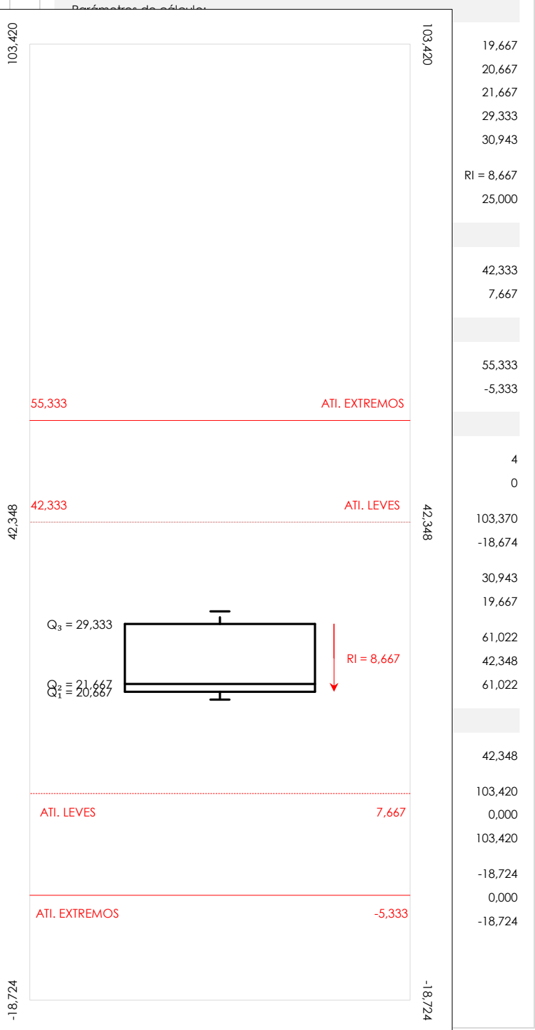
Diagrama Box-Plot post-estadístico. Eje Y: prof.maxim.penet.agua hormigon (mm)
