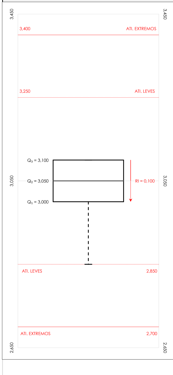
Diagrama Box-Plot post-estadístico. Eje Y: contenido aire (%)
