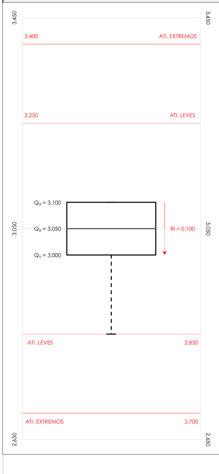
Diagrama Box-Plot pre-estadístico. Eje Y: contenido aire (%)
