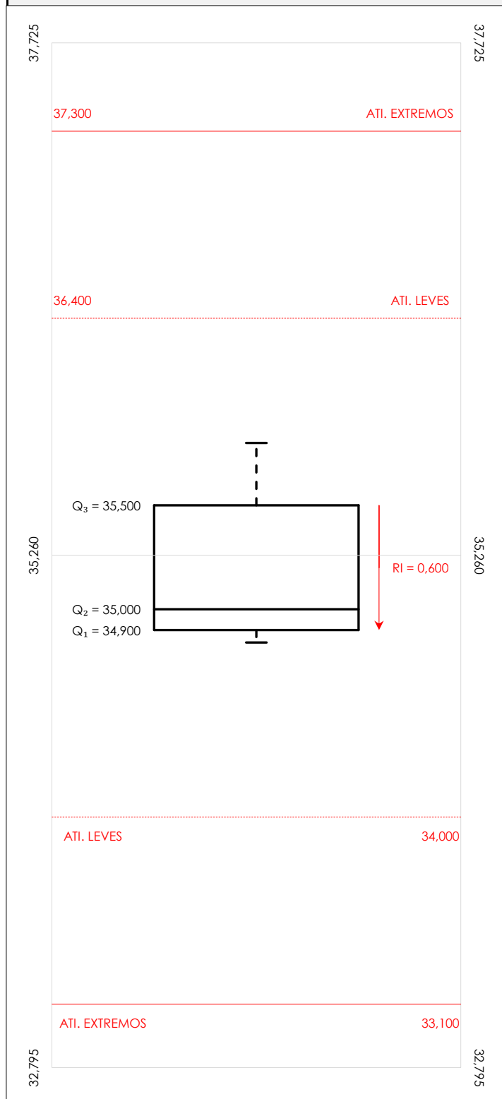
Diagrama Box-Plot post-estadístico. Eje Y: dnt Ais.Acústic.Aéreo fr1000 hz (dB)
