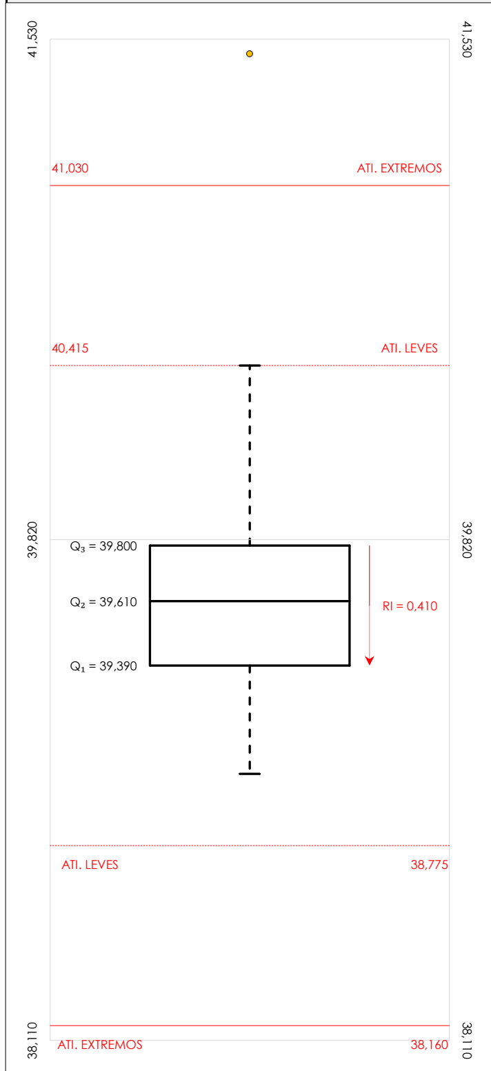
Diagrama Box-Plot pre-estadístico. Eje Y: dnt Ais.Acústic.Aéreo fr1600 hz (dB)
