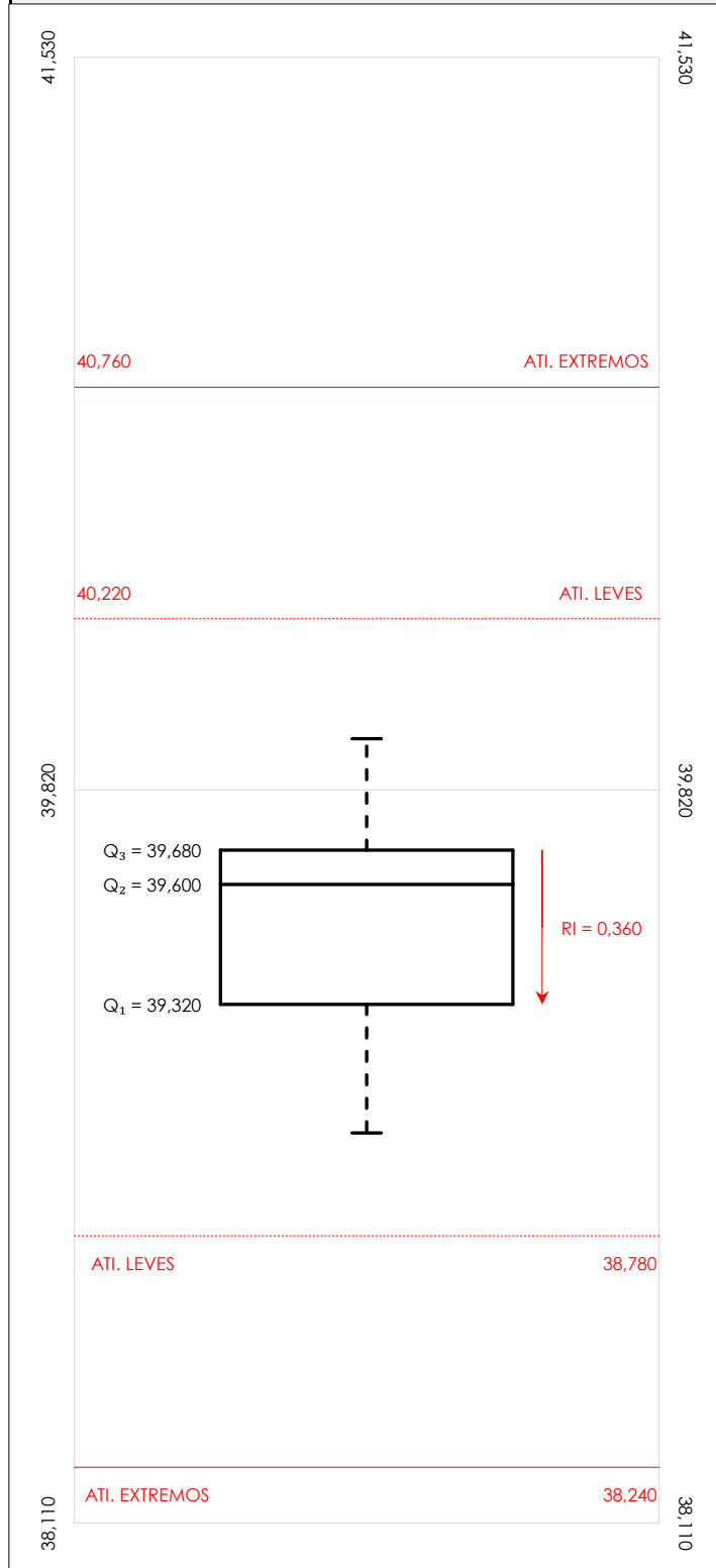
Diagrama Box-Plot post-estadístico. Eje Y: dnt Ais.Acústic.Aéreo fr1600 hz (dB)
