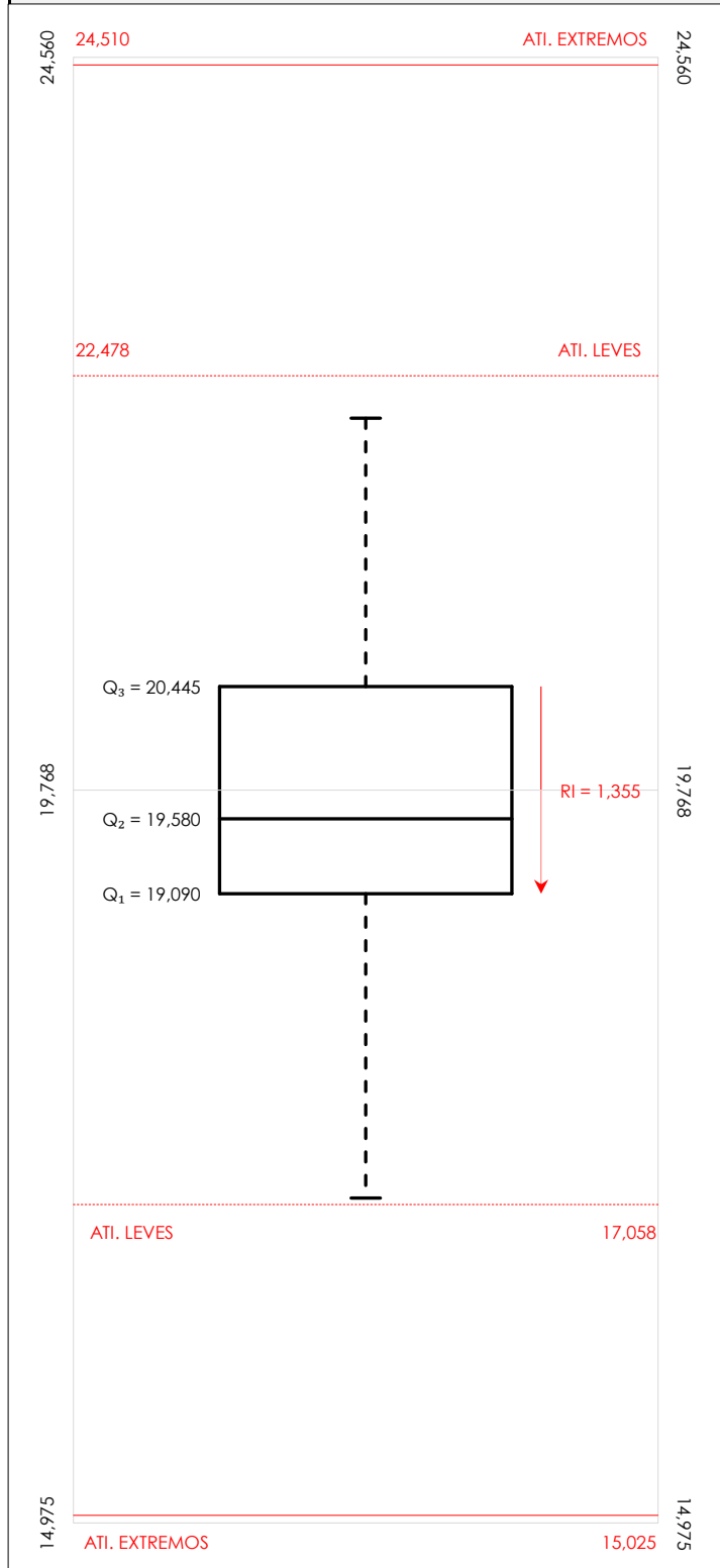
Diagrama Box-Plot pre-estadístico. Eje Y: dnt Ais.Acústic.Aéreo fr125 hz (dB)
