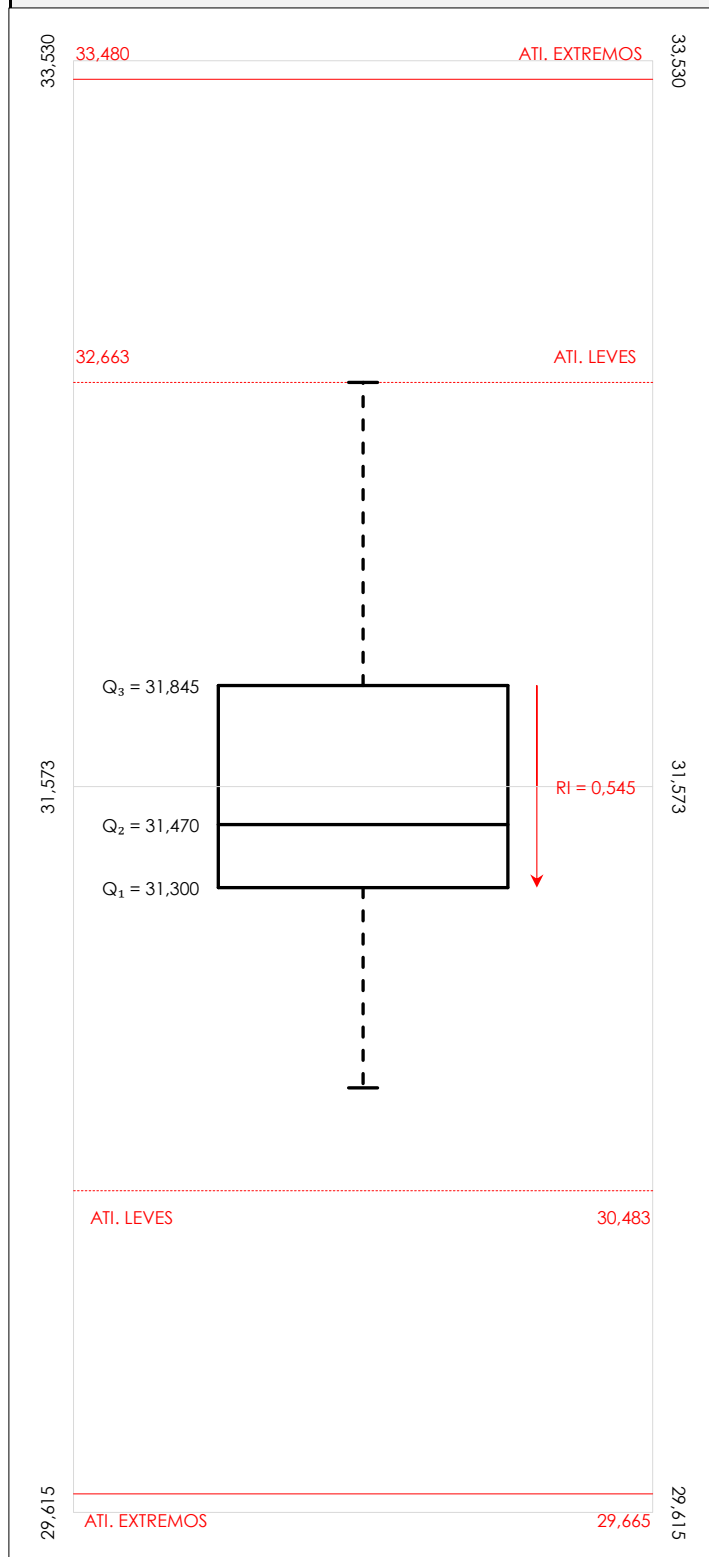
Diagrama Box-Plot post-estadístico. Eje Y: dnt Ais.Acústic.Aéreo fr400 hz (dB)
