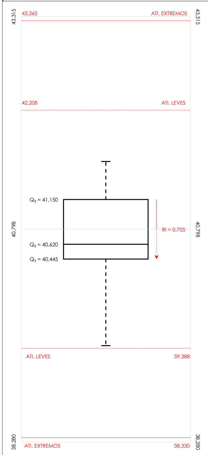
Diagrama Box-Plot pre-estadístico. Eje Y: dnt Ais.Acústic.Aéreo fr3150 hz (dB)
