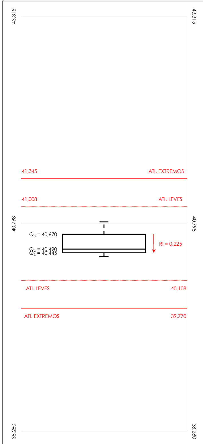
Diagrama Box-Plot post-estadístico. Eje Y: dnt Ais.Acústic.Aéreo fr3150 hz (dB)
