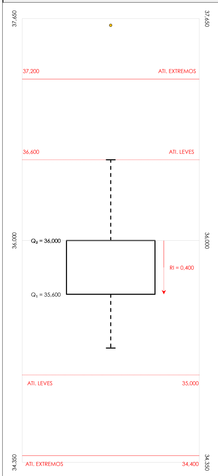
Diagrama Box-Plot pre-estadístico. Eje Y: dnt w valor global (dB)
