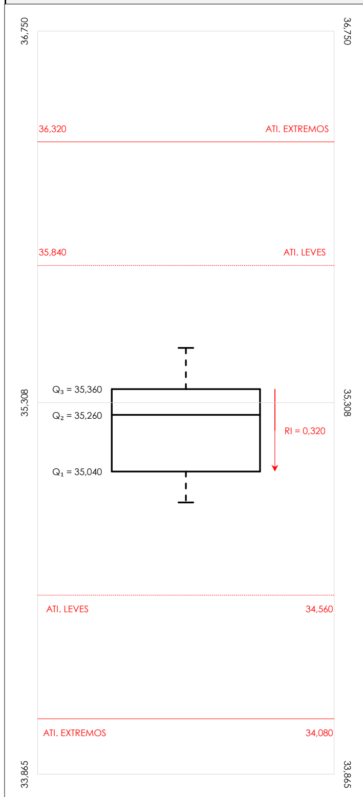
Diagrama Box-Plot post-estadístico. Eje Y: dnt Ais.Acústic.Aéreo fr800 hz (dB)
