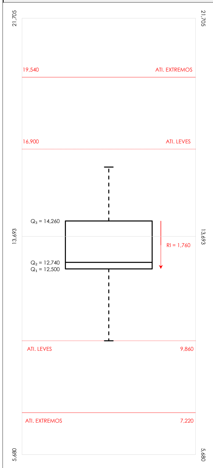
Diagrama Box-Plot post-estadístico. Eje Y: dnt Ais.Acústic.Aéreo fr100 hz (dB)
