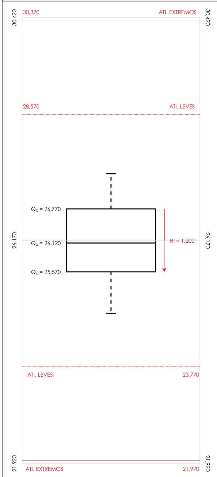
Diagrama Box-Plot post-estadístico. Eje Y: dnt Ais.Acústic.Aéreo fr160 hz (dB)
