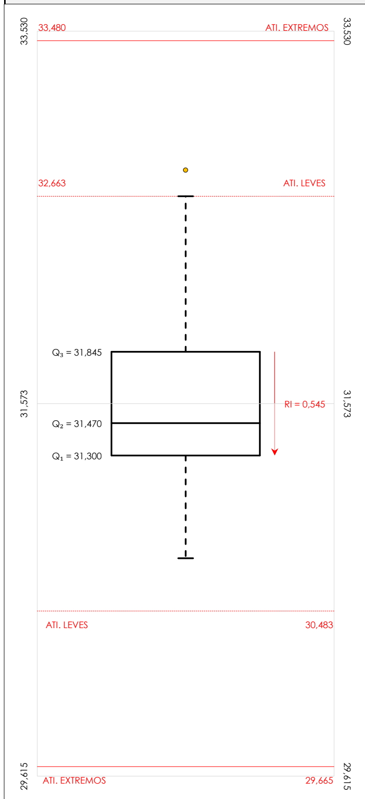
Diagrama Box-Plot pre-estadístico. Eje Y: dnt Ais.Acústic.Aéreo fr400 hz (dB)
