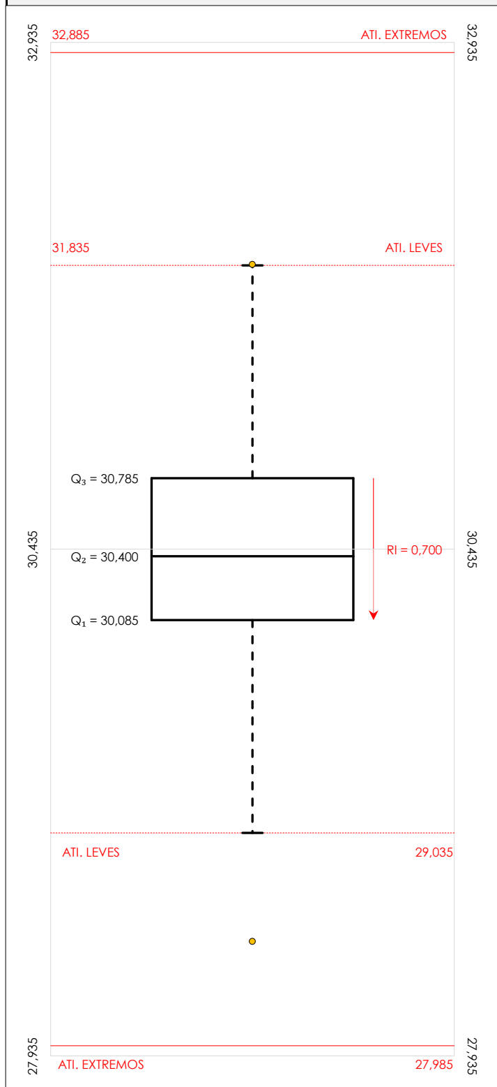
Diagrama Box-Plot pre-estadístico. Eje Y: dnt Ais.Acústic.Aéreo fr315 hz (dB)
