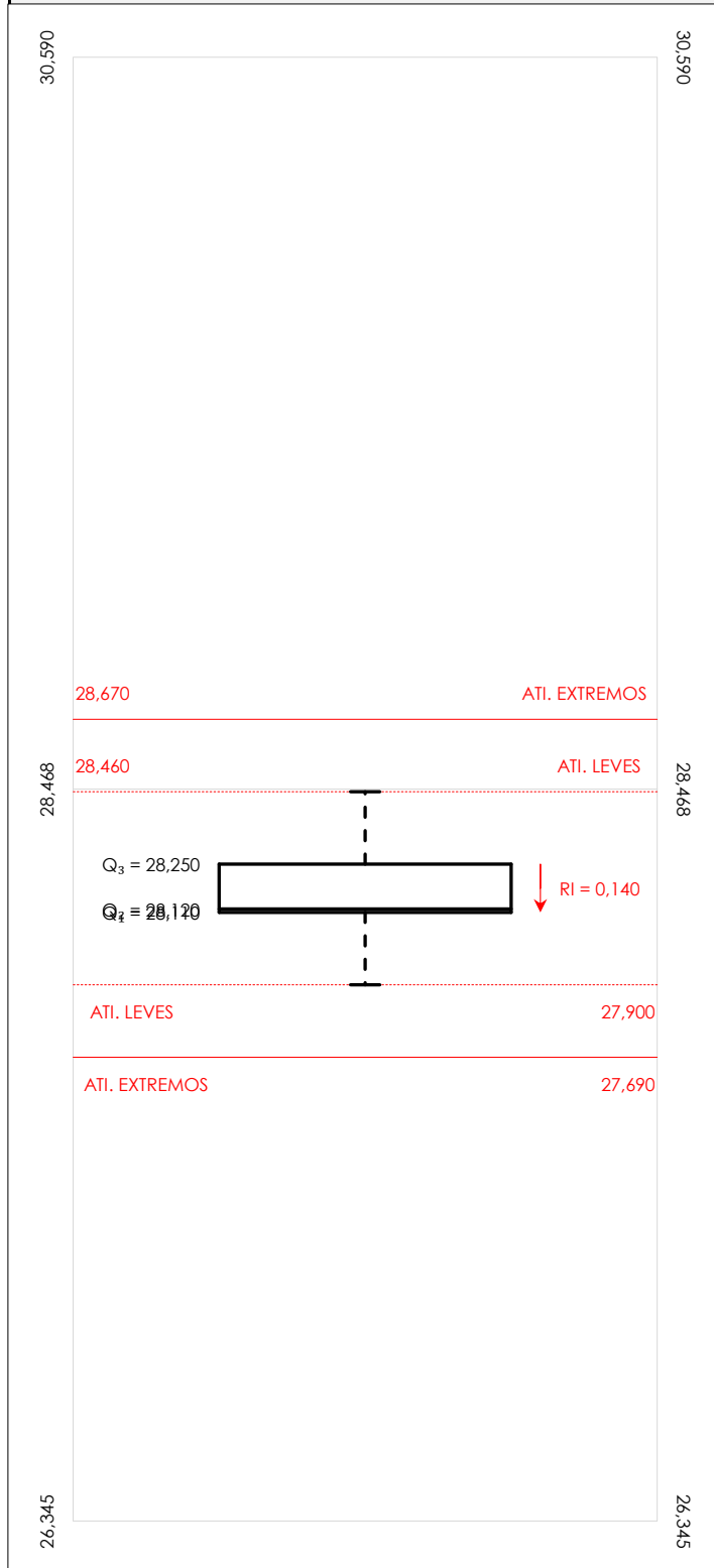
Diagrama Box-Plot post-estadístico. Eje Y: dnt Ais.Acústic.Aéreo fr200 hz (dB)
