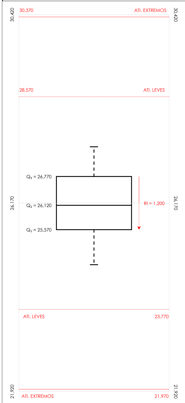
Diagrama Box-Plot pre-estadístico. Eje Y: dnt Ais.Acústic.Aéreo fr160 hz (dB)
