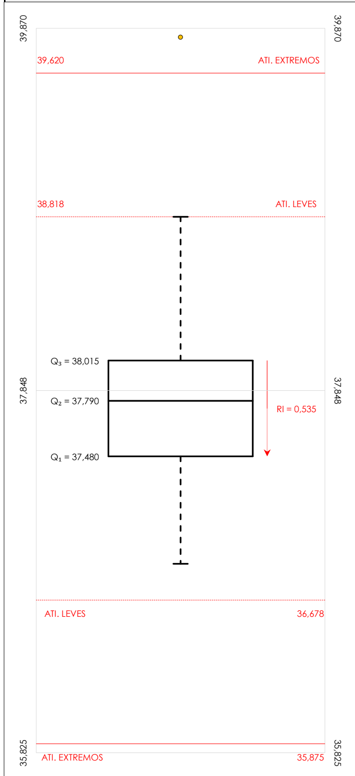
Diagrama Box-Plot pre-estadístico. Eje Y: dnt Ais.Acústic.Aéreo fr1250 hz (dB)
