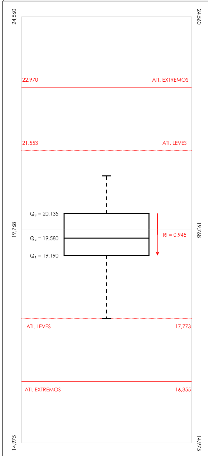
Diagrama Box-Plot post-estadístico. Eje Y: dnt Ais.Acústic.Aéreo fr125 hz (dB)
