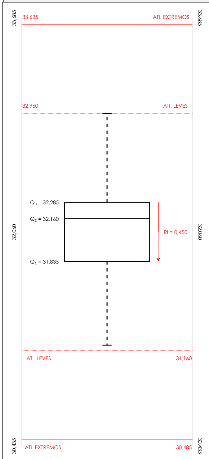
Diagrama Box-Plot post-estadístico. Eje Y: dnt Ais.Acústic.Aéreo fr500 hz (dB)
