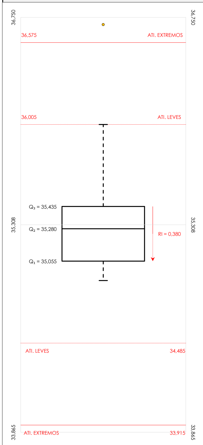
Diagrama Box-Plot pre-estadístico. Eje Y: dnt Ais.Acústic.Aéreo fr800 hz (dB)
