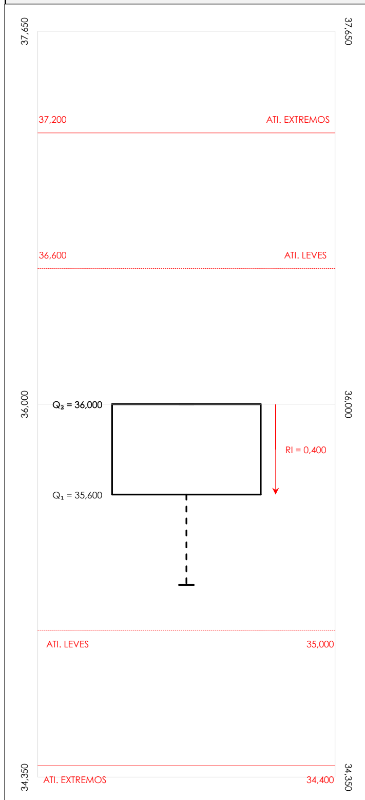
Diagrama Box-Plot post-estadístico. Eje Y: dnt w valor global (dB)
